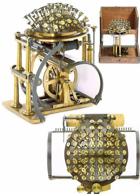
Pastor R. Malling-Hansens Skrivekugle af nyeste Construction.
